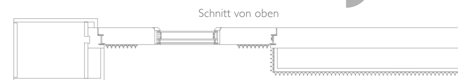
CHICAGO EDGEWATER mit Chicago-Verblendung RAL 8029 / ES s 204 / U_g : 0,71
